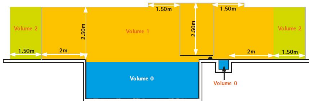
Dimensions des volumes pour piscines et pédiluves.
