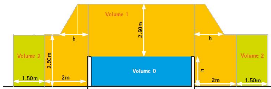
Dimensions des volumes pour piscines hors sol
